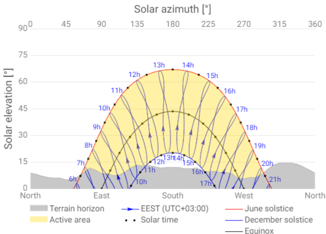
Diagrama de poziție a soarelui pe cer specifică zonei Orașului Baia de Arieș ( globalsolaratlas.info )
